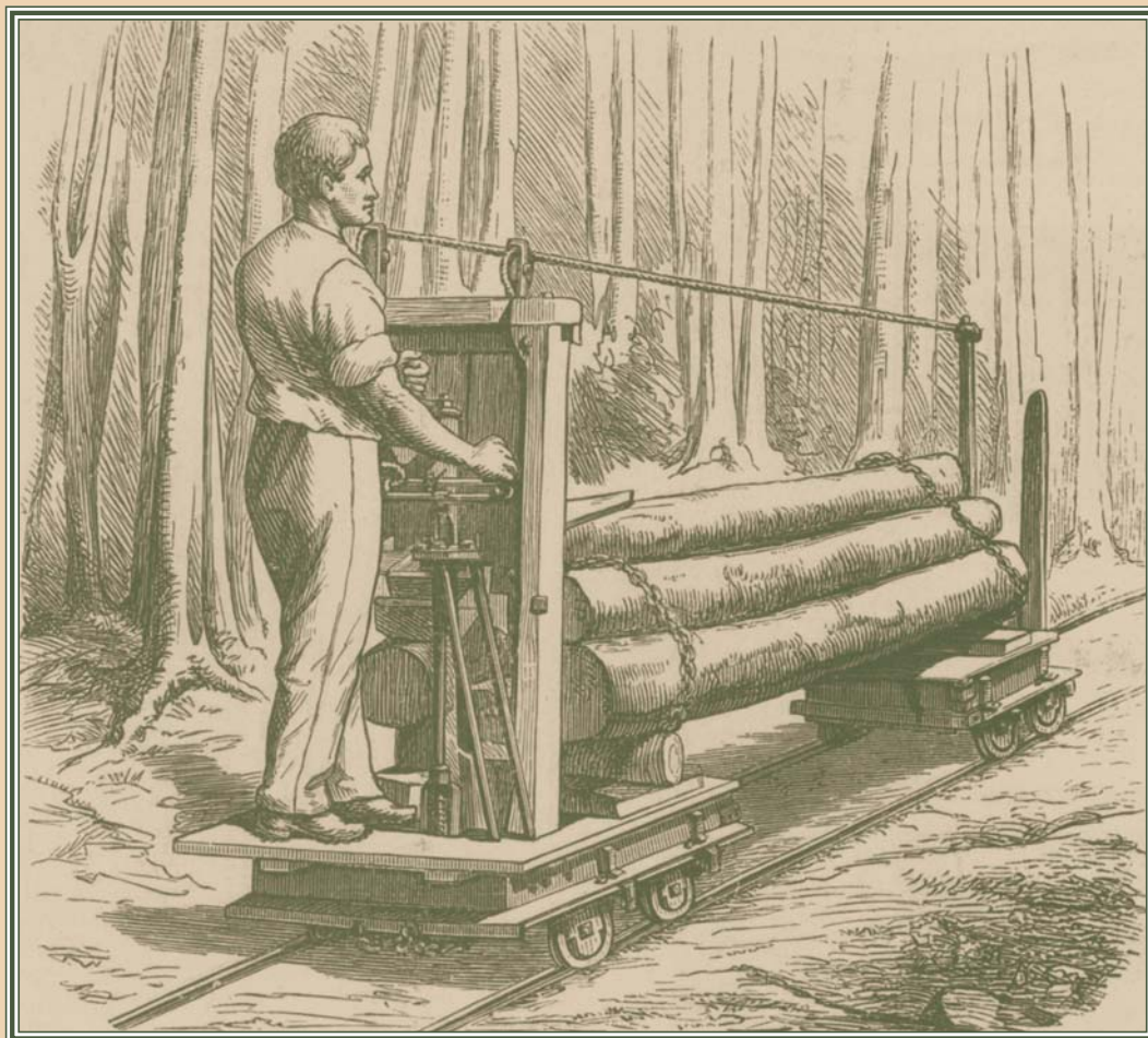
Kolejová doprava dřeva po mírném svahu ( K. Gayer, H. Mayr, Die Forstbenutzung, 1909 ).
